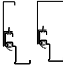
Umfassungszarge 2-schalig Zargenspiegel 33 mm oder 76 mm
