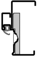
Universal-Eckzarge mit Ergänzungszarge Vario B53
